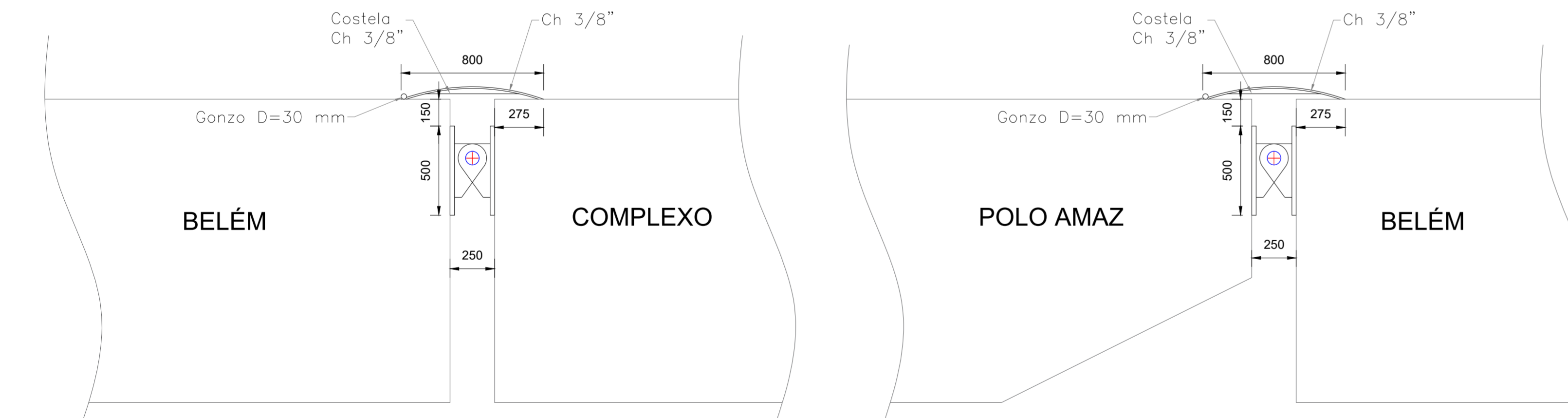
VISTA SUPERIOR - CHAPA DE CONEXÃO BELÉM - COMPLEXO
