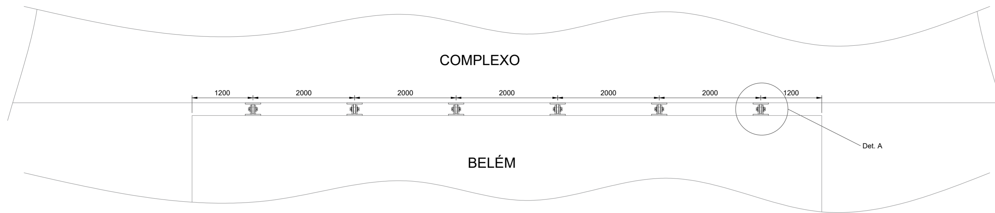
VISTA SUPERIOR - POSIÇÃO OLHAIS DE CONEXÃO E CHAPA PARA PASSAGEM DE VEÍCULOS
