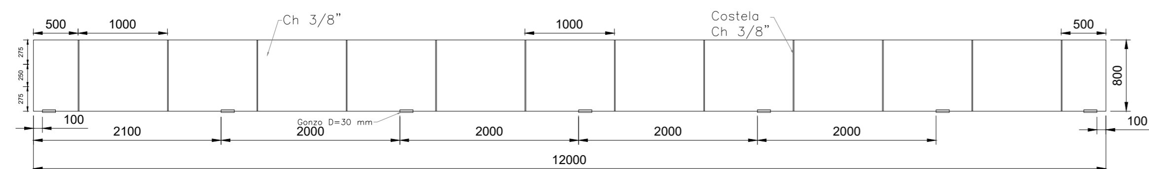
VISTA SUPERIOR - CHAPA DE CONEXÃO BELÉM - POLO AMAZ.
