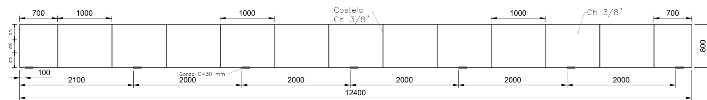
VISTA SUPERIOR - CHAPA DE CONEXÃO BELÉM - POLO AMAZ.
